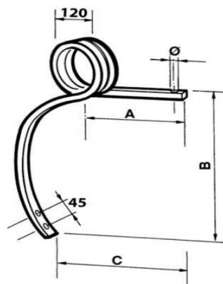
Il disegno rappresenta una molla sinistra
